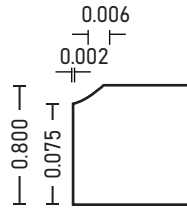
DETALLE SENEFA
